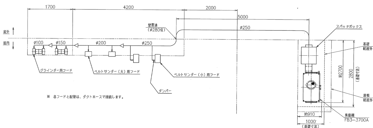
全体集塵装置図
